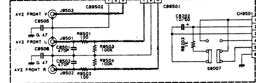
AV FRONT P. C. Board
