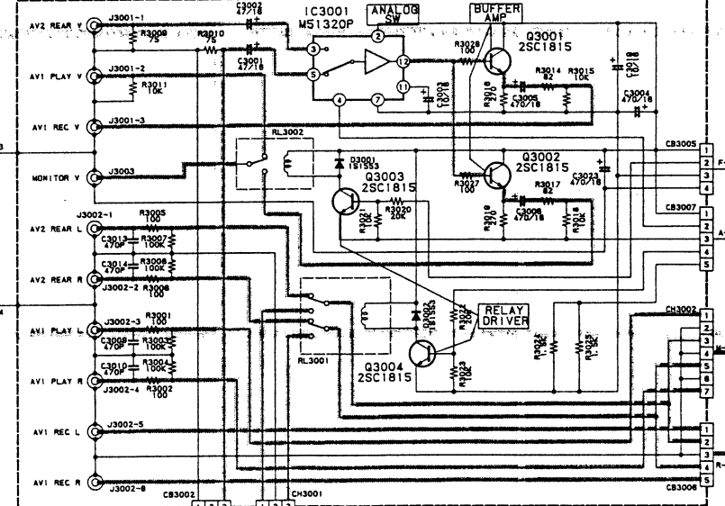
AV FRONT P. C. Board
